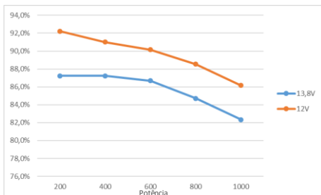
Rendimento % - 1000W-12E220S X Potência de saída
