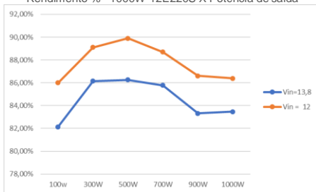
Rendimento % - 1000W-12E220S X Potência de saída
